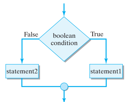
If-else syntax
